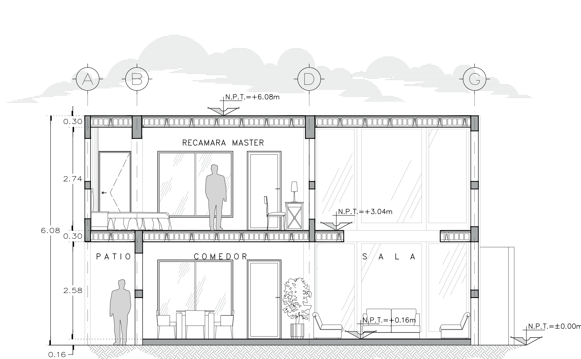
CORTE TRANSVERSAL X-X' ESCALA 1:50
