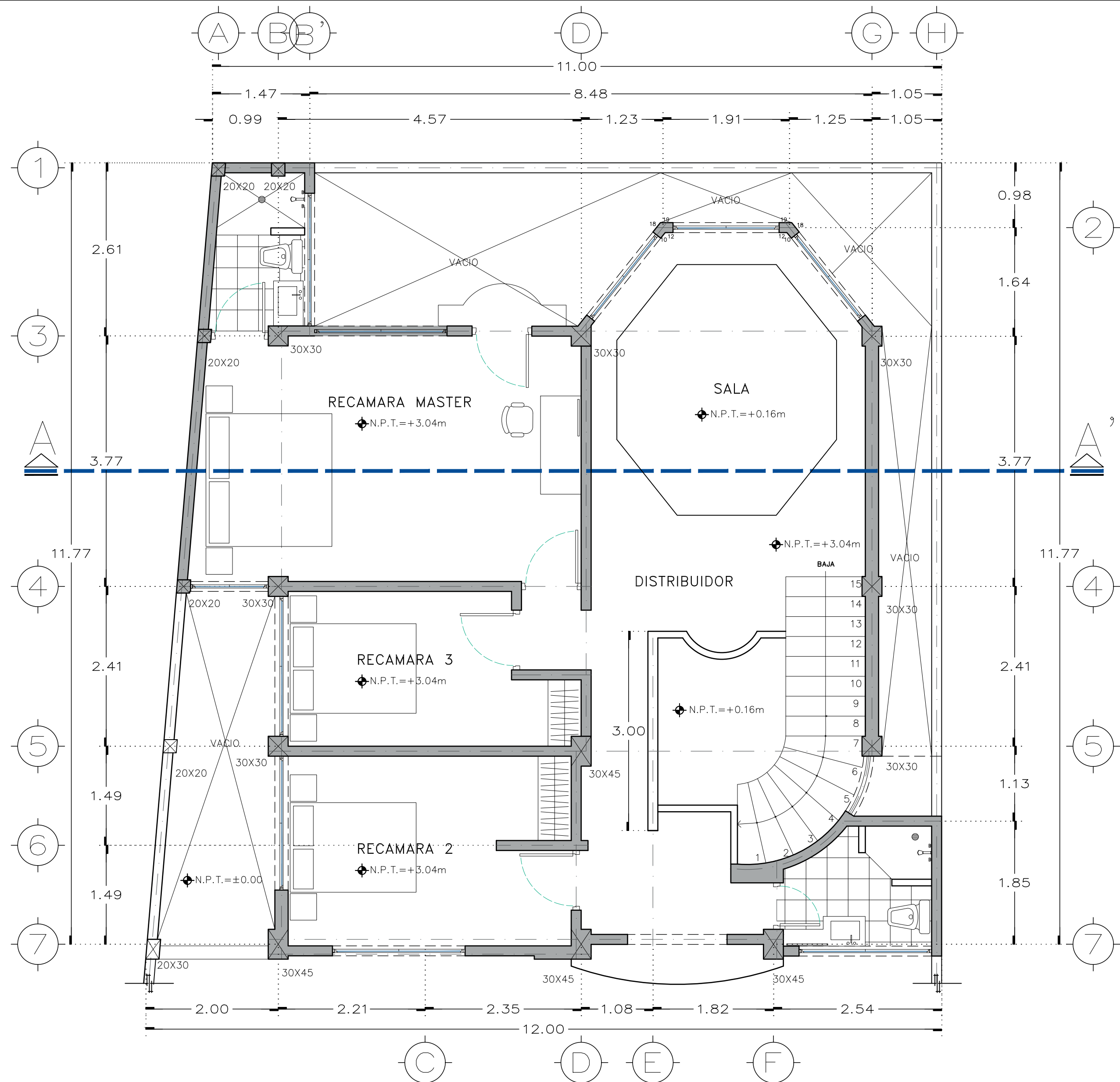
PLANTA ARQUITECTONICA ALTA ESCALA 1:50
