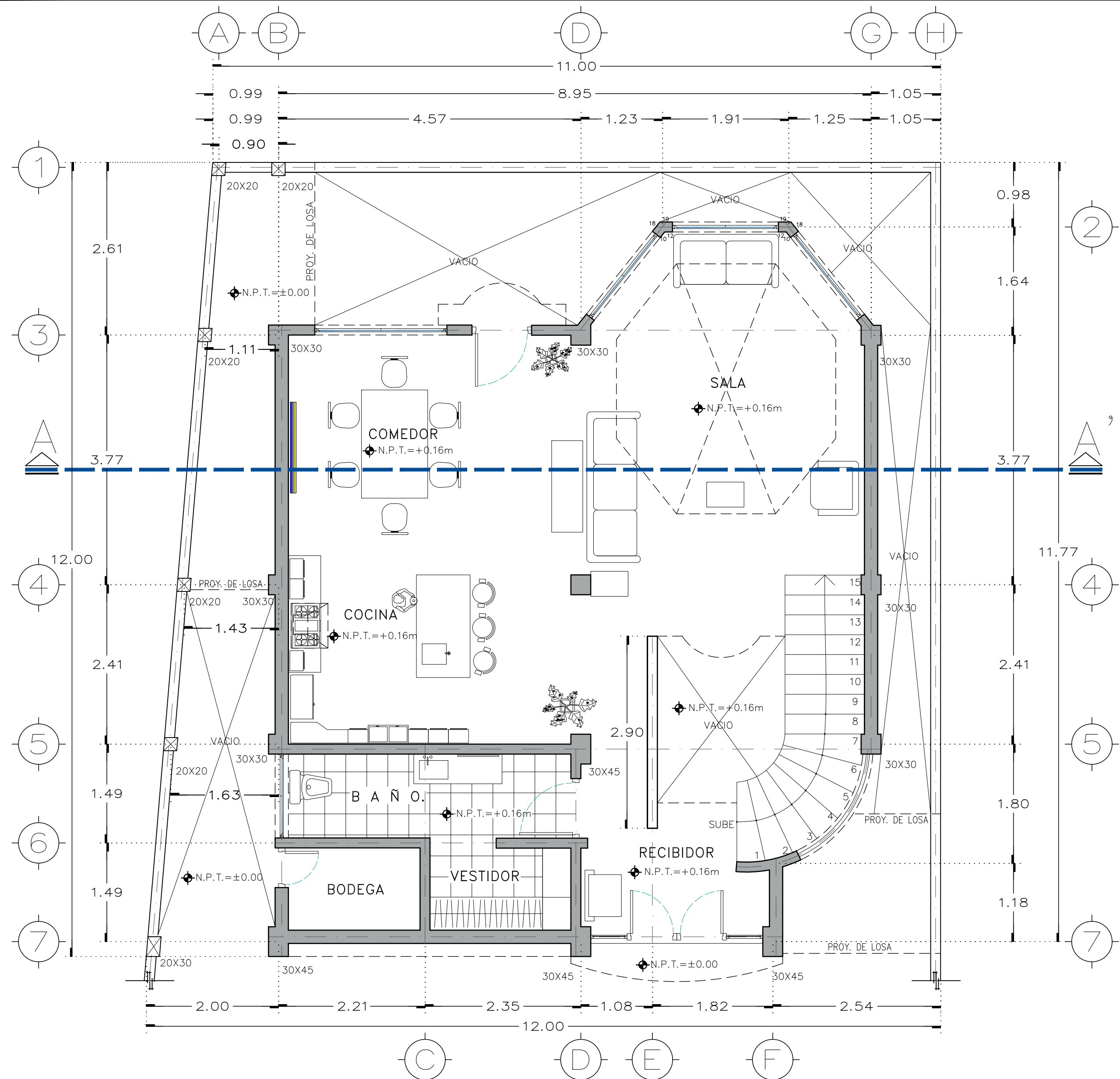
PLANTA ARQUITECTONICA BAJA ESCALA 1:50
